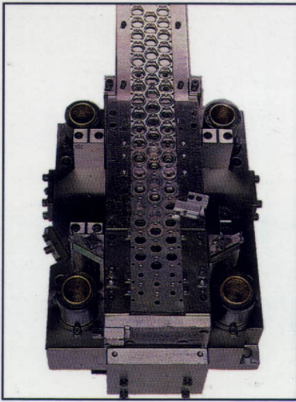
TAB DIE
